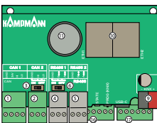
Draufsicht Mainboard
