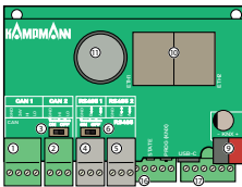
Vue de dessus de la carte mère
